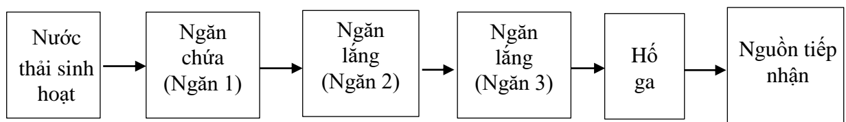
Hình 7 – Quy trình xử lý nước thải sinh hoạt
