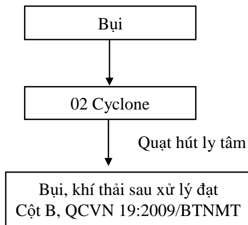
Hình 9. Sơ đồ xử lý bụi tại công đoạn xay bóc vỏ
